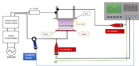
รูปที่ 1 เครื่องกำเนิดพลาสมาโคโรนาดีสชาร์จแบบมีฉนวนกัน
