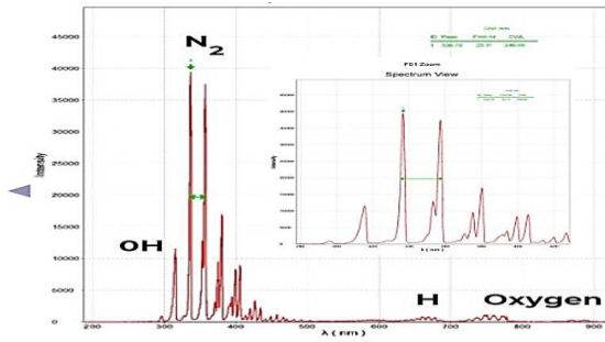
รูปที่ 3 สเปกโทรสโกปีการปล่อยแสง (The optical emission spectroscopy, OES) ของพลาสมาโพลิเอทิลีนที่ผ่านการบำบัดด้วยพลาสมา
